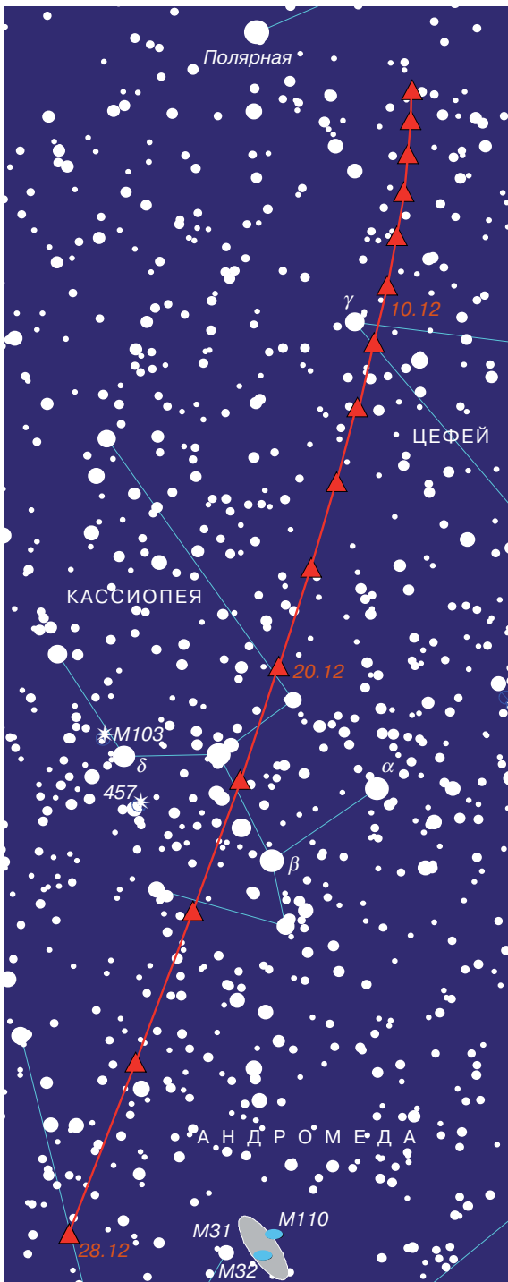
Комета 8P/Tuttle в декабре 2007 г.
