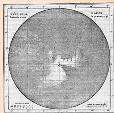
Зарисовки туманности Ориона, опубликованные Мессье в первой версии его знаменитого каталога в Трудах Королевской Академии (Memoires de l'Academie Royale) в 1771 г.
