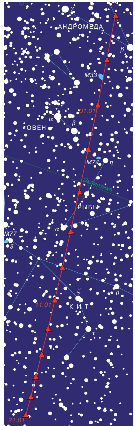
8P/Tuttle в начале 2008 г.
