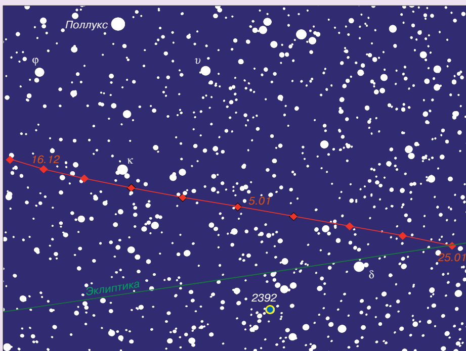
Путь астероида Евномия (15 Eunomia) по созвездию Близнецов в декабре 2007 — январе 2008 г.
