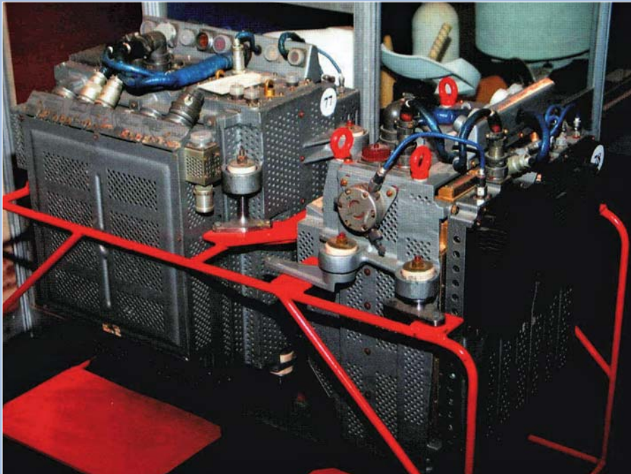
Общий вид аппаратуры системы стыковки "Игла".
