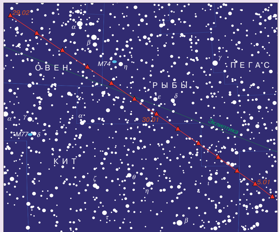
Комета 46P/Wirtanen на вечернем небе в январе-феврале 2008 г.
